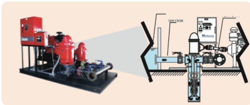
Equipo con motobombas tipo turbinas verticales.
