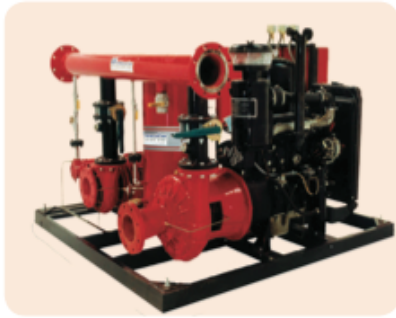
Equipo para gastos de hasta 1,000 gls/min.
